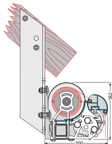
Dachsparren
