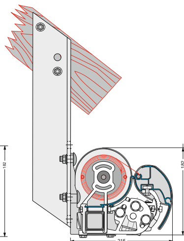
Dachsparren
