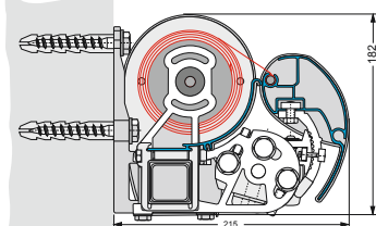
Wand
