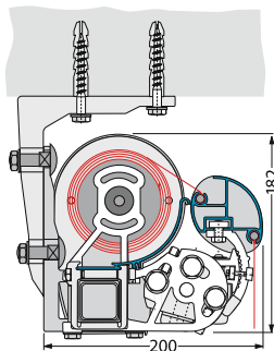
Decke
