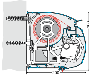
Wand
